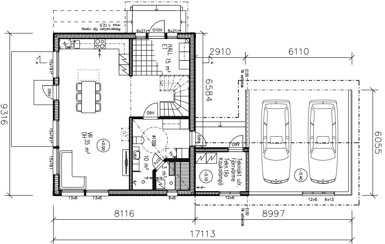
Plan, vån 1
