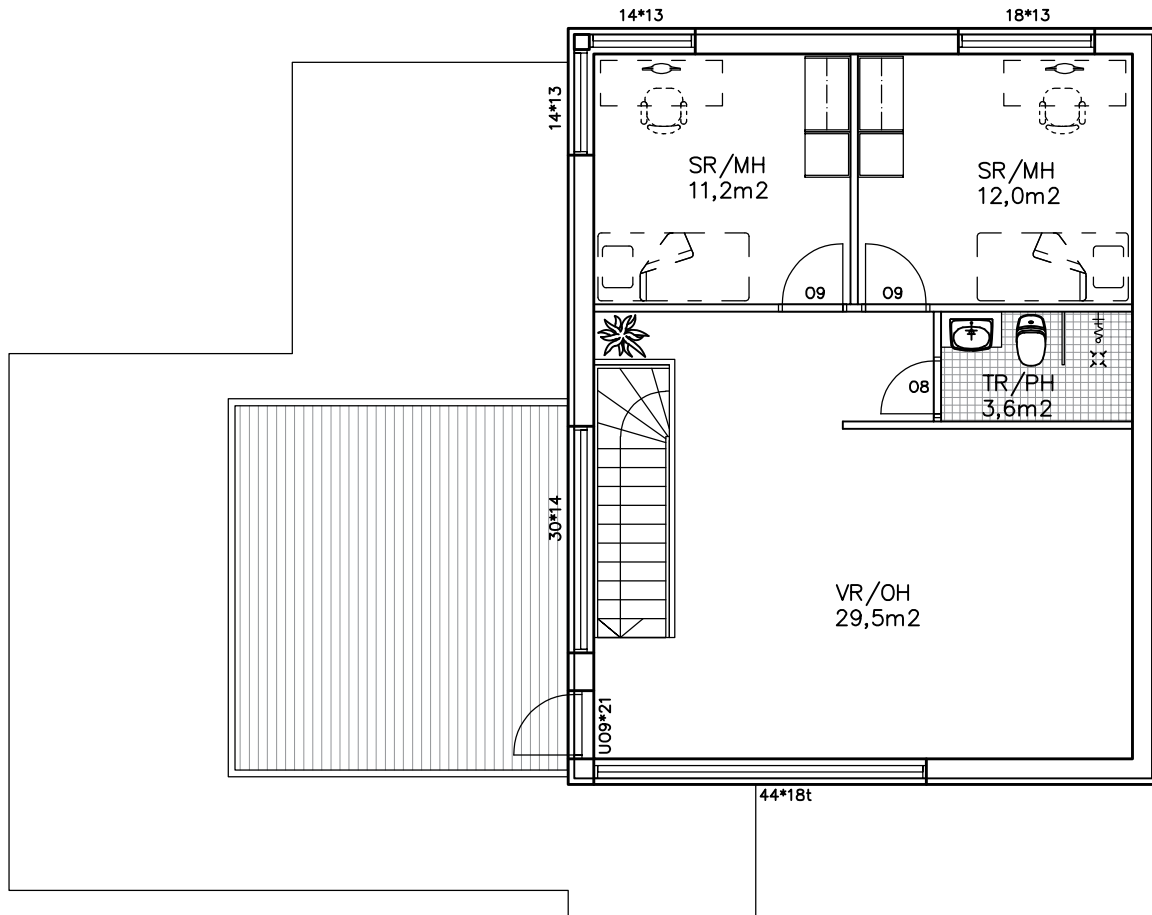
Våning 2 / Kerros 2
