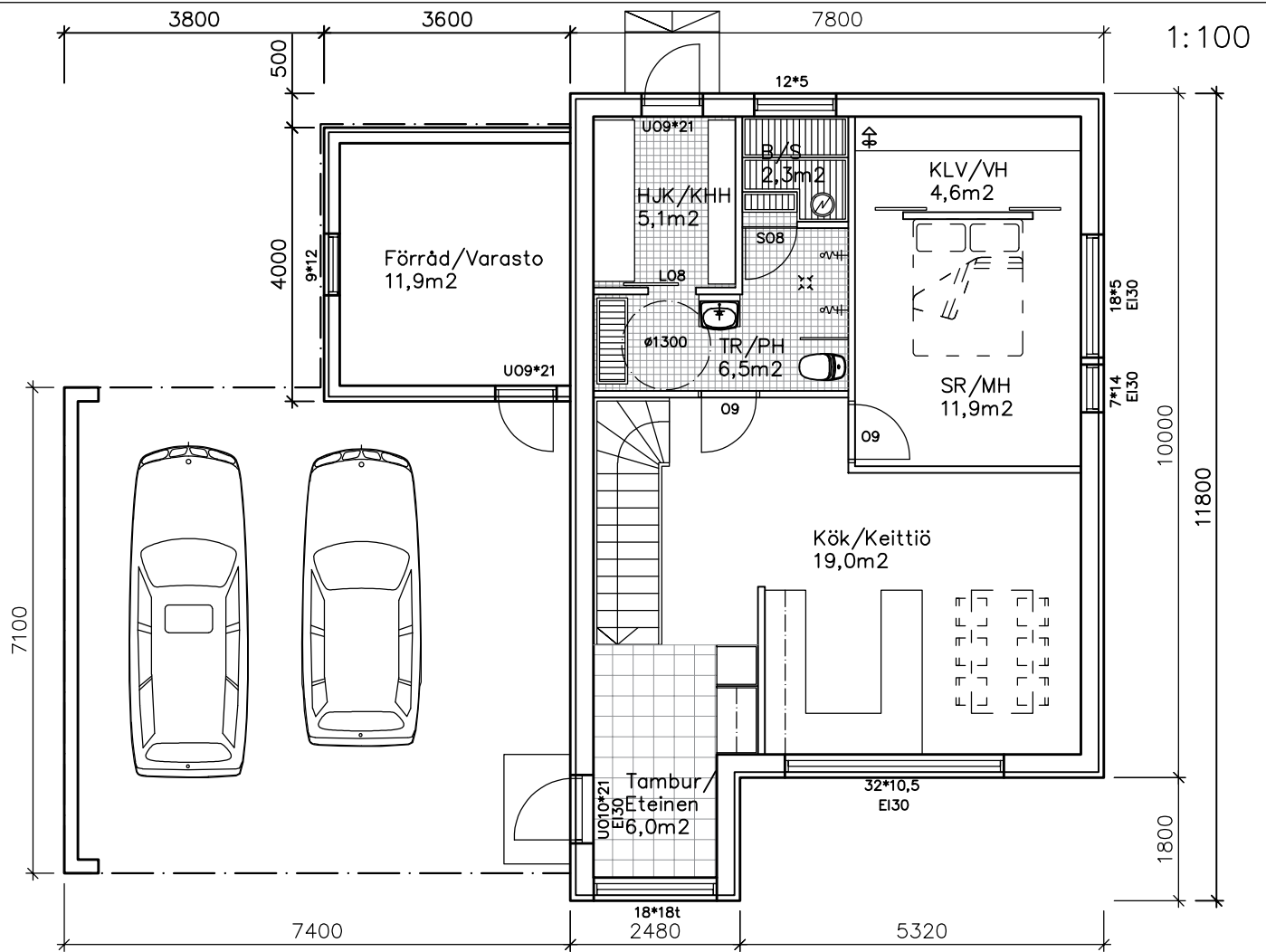
Våning 1 / Kerros 1
