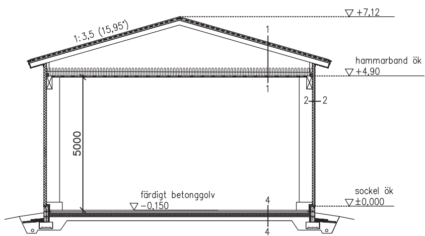
SKÄRNING A-A
